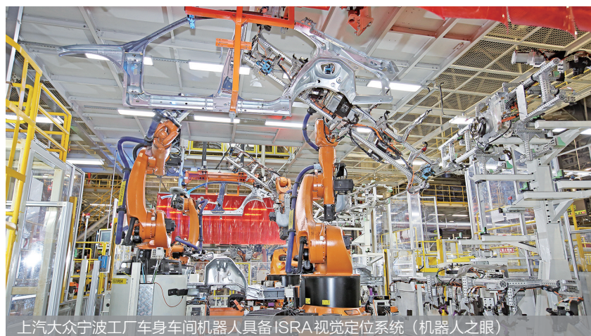
上汽大众宁波工厂车身车间机器人具备ISRA视觉定位系统（机器人之眼）
