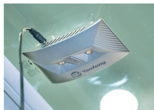
车规级深紫外线杀菌盒，工作10分钟即可完成对内表面的杀菌，实现99%的病毒灭活率
